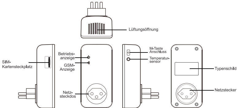
Abbildung 1: SMS-Butler-Mobile Bedienelemente und Funktionen
