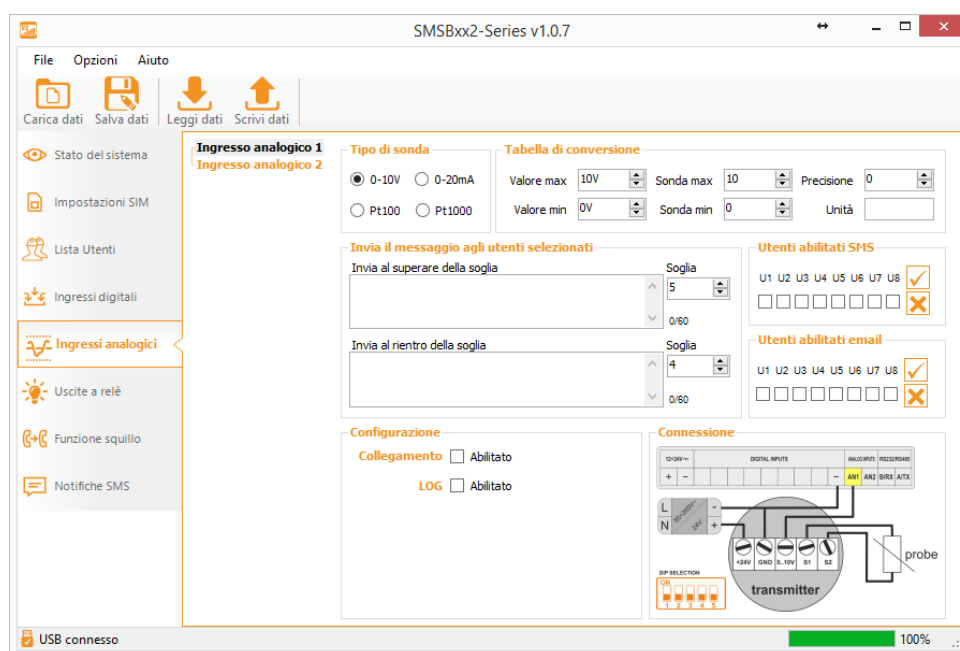
Figura 5: Ingressi analogici
